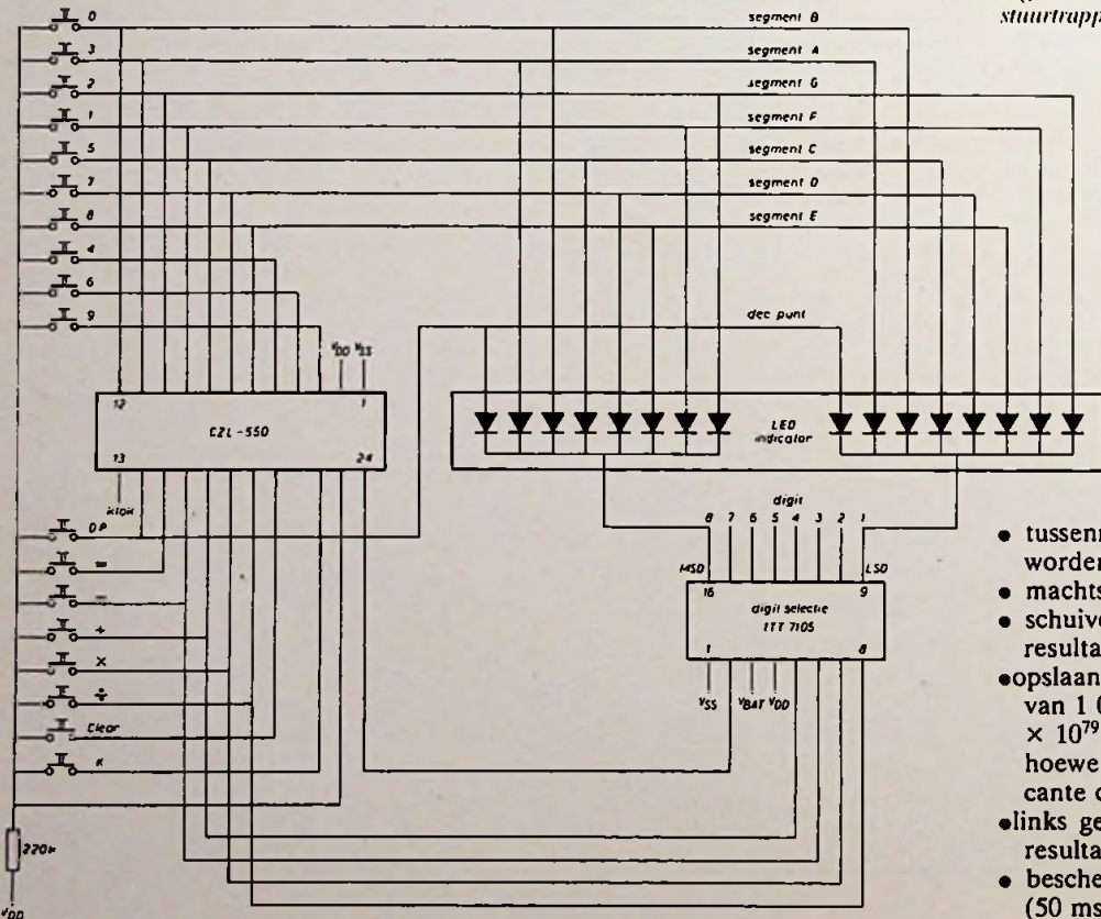
Fig. 2. Een eenvoudige calculator met de CZL-550.
